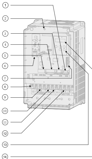
图 1-2 伺服驱动器组成
