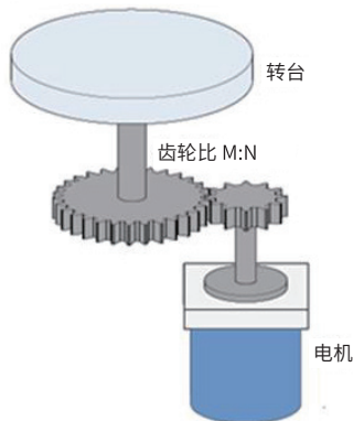
图 4-13 旋转负载示意图
