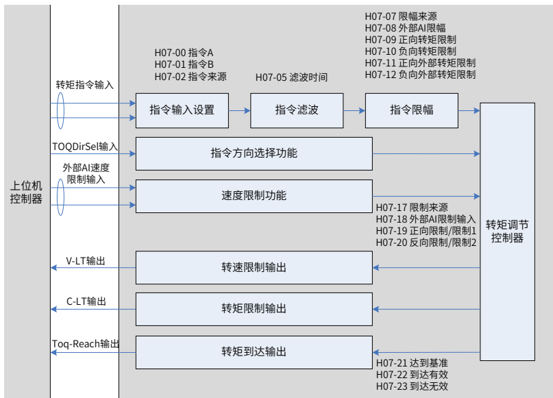
图 4-10 转矩控制模式框图
