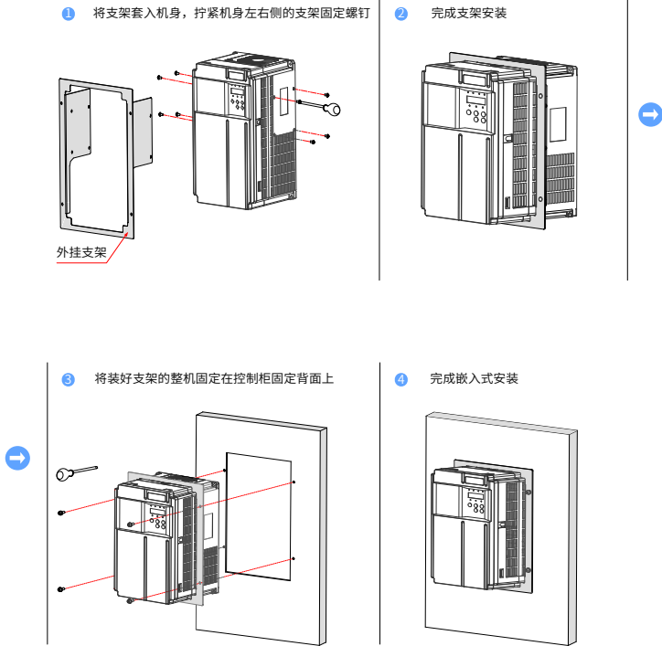
图 2-10 IS650PT025IUX-B、IS650PT032IUX-B、IS650PT037IUX~IS650PT060IUX 机型嵌入式安装示意图
