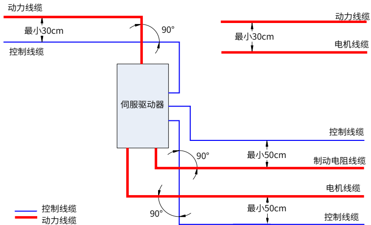
图 3-37 电缆布线图
