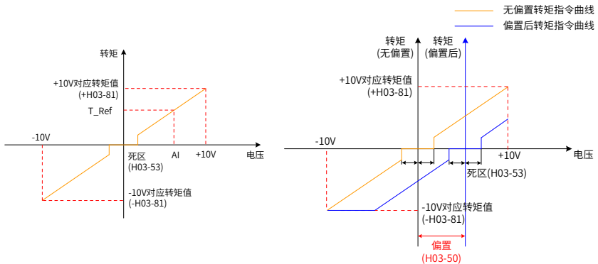
无偏置 AI1 示意图
