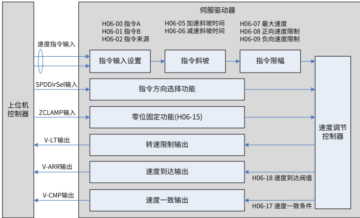
图 4-5 速度控制模式框图
