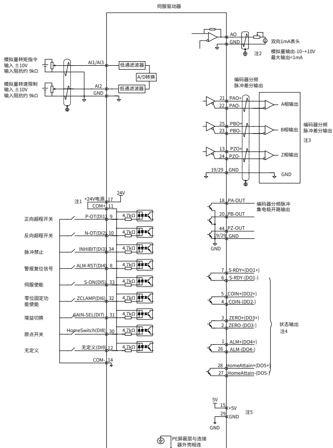
图 4-11 转矩模式配线图
