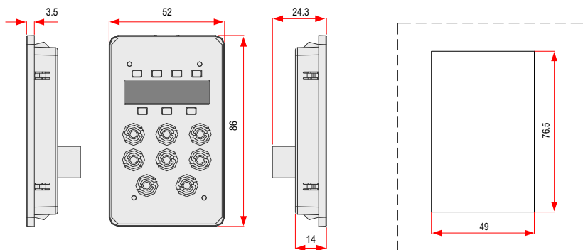
图 D-3 MD310-KEY1 外引键盘安装尺寸图 (单位: mm)
