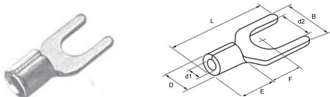
图 3-12 TNS 系列叉形线耳外观及尺寸图（【注】）
