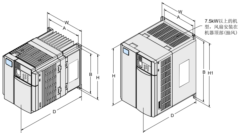
0.4kW-2.2kW 外形及安装尺寸示意图
