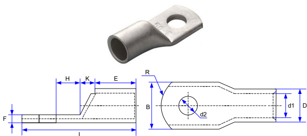
图 3-10 GTNR 系列圆型线耳外观及尺寸图 (推荐)
