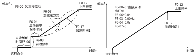
图 4-9 直接启动方式
