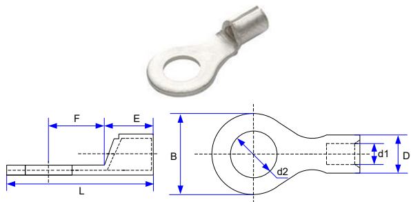
图 3-11 TNR 系列圆型线耳外观及尺寸图 (推荐)
