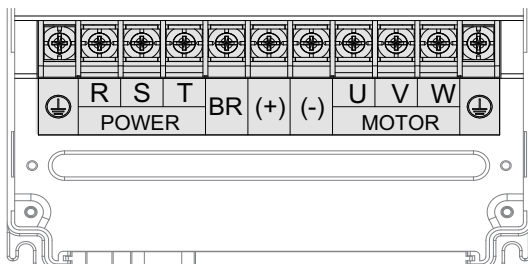
图2-4 T5~T8机型主回路端子分布图
