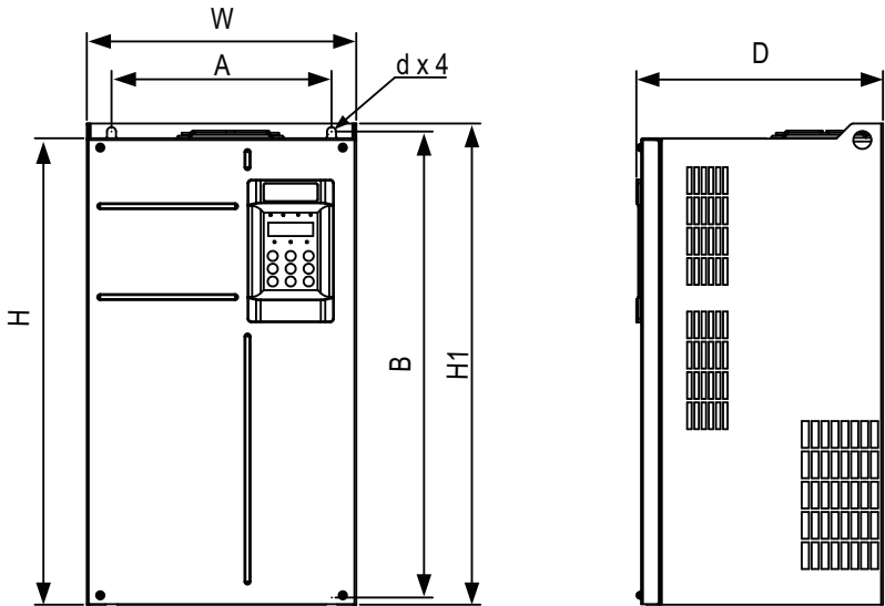
图1-3 T7~T9外型尺寸及安装尺寸示意图
