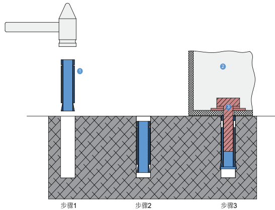
图1-20 膨胀螺钉安装示意图
