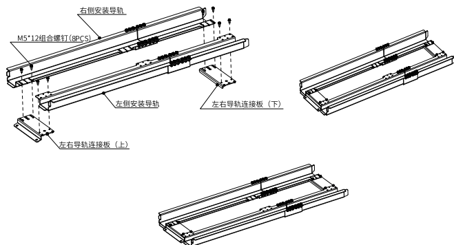
图1-12 安装导轨组装示意图
