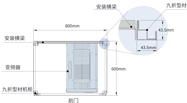
图1-9 T11~T12机型机柜俯视图
