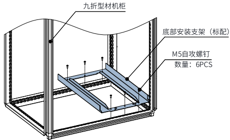
图1-11 底部安装支架安装示意图
