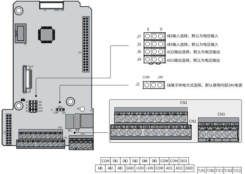
图2-8 控制回路端子分布图
