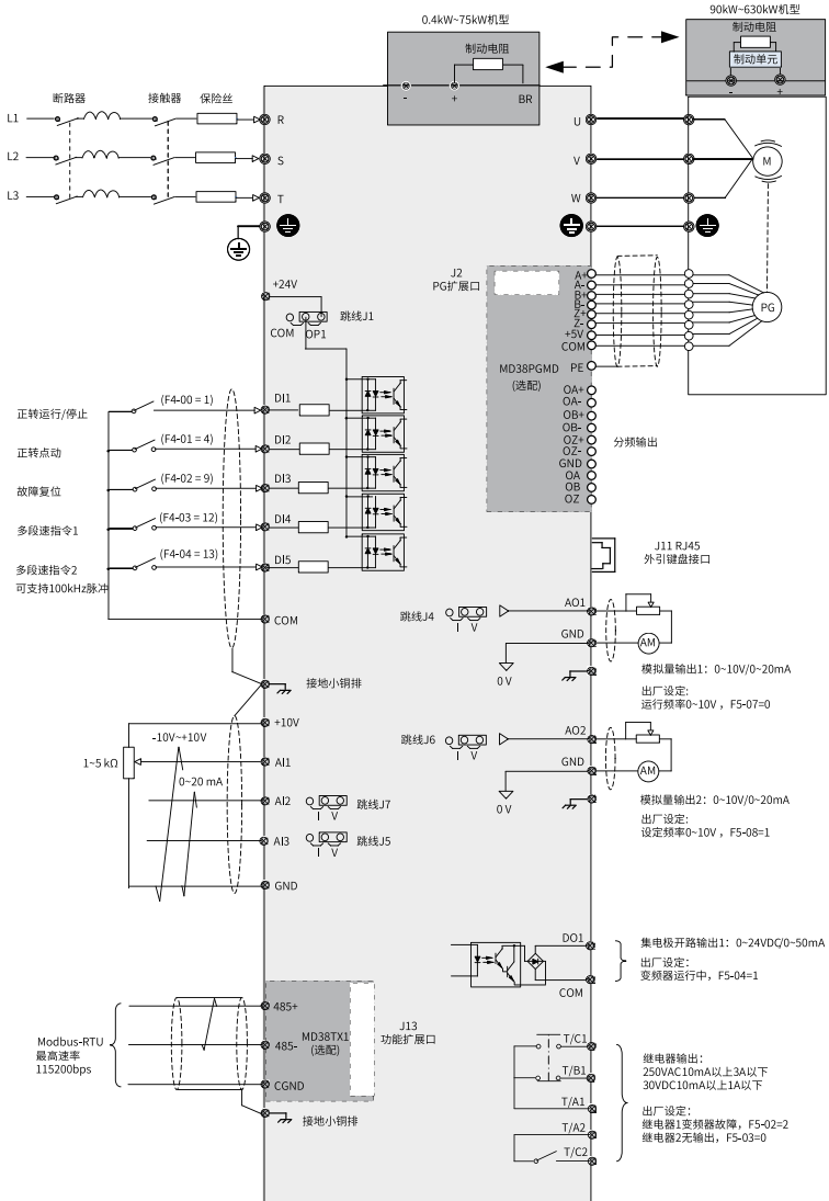
图2-1 标准接线图
