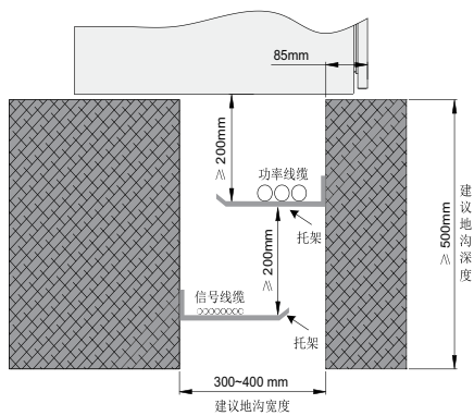
图1-21 地基布局图
