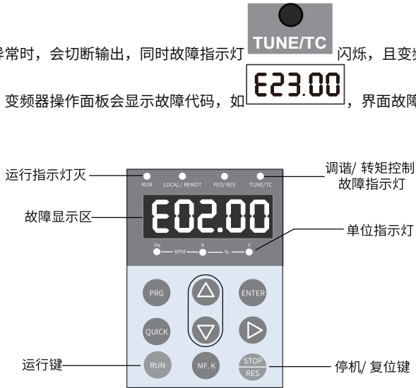
图4-1 界面故障显示
